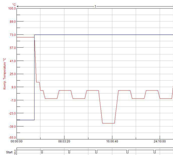
Рисунок А.1 – Графическая модель одного цикла климатических испытаний
