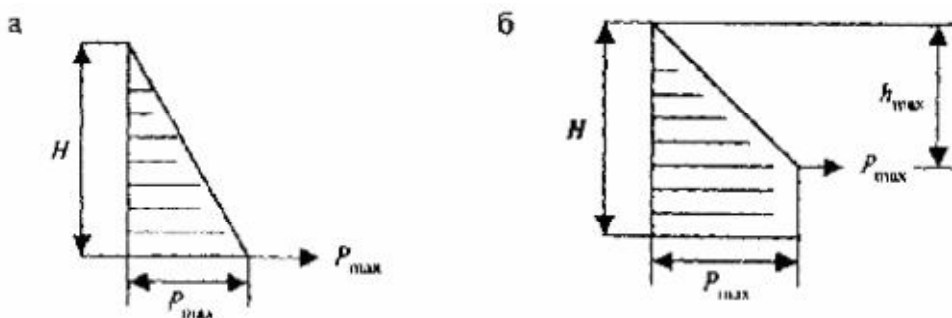
Рисунок 16.1 Расчетные эпюры бокового давления бетонной смеси
