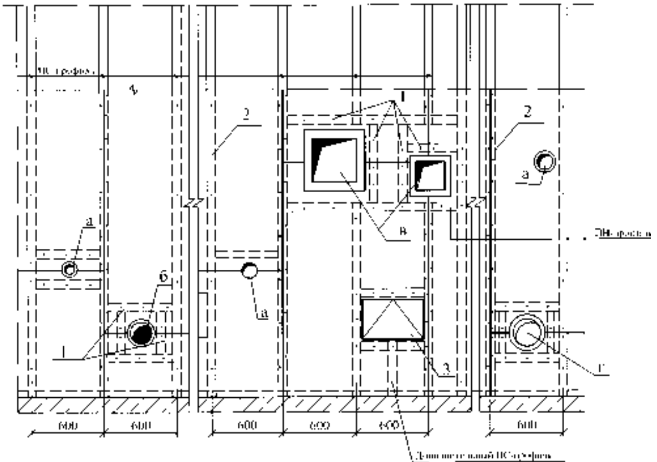
Рисунок 5 — Схема размещения трубопроводов диаметром не более 60 мм (а), технологических трубопроводов — не менее 60 мм (б), воздухопроводов (в) и трубопроводов водоснабжения и отопления (г)
