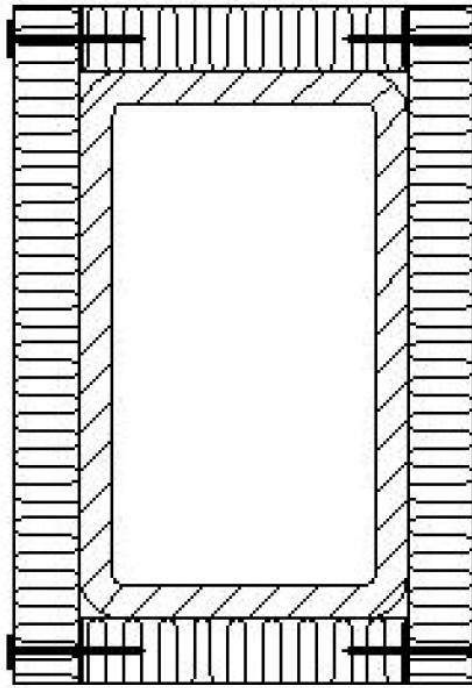
Рисунок 5.5. Схема покрытия по поверхности металлической конструкции прямоугольного сечения.
